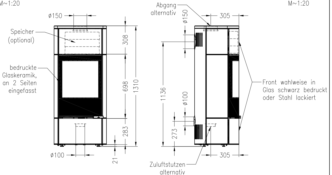
Draufsicht M~1:10
